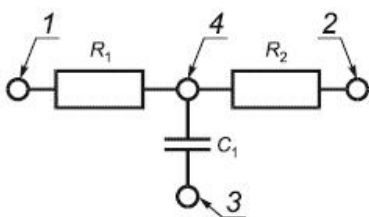
Рисунок В.1 - Составная мера активного сопротивления и емкости
